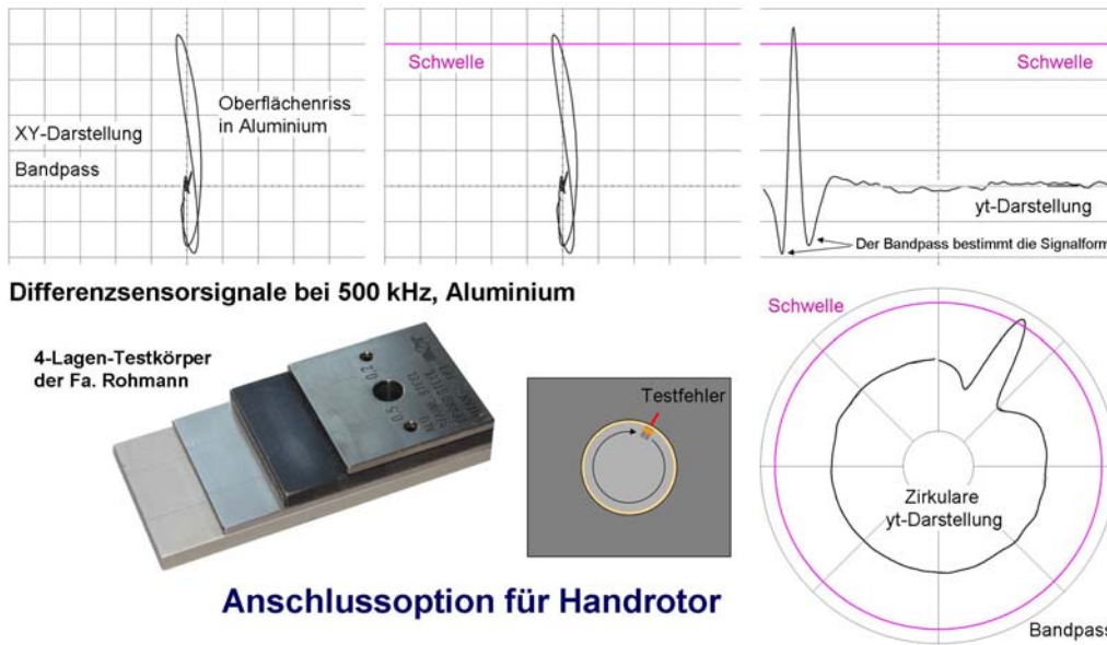
Bild 6: Signale eines Innenrotiersensors (Differenzsensor)
