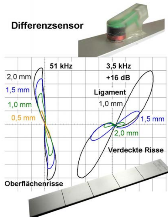
Bild 4: Rissprüfung mit dem Differenzsensor
